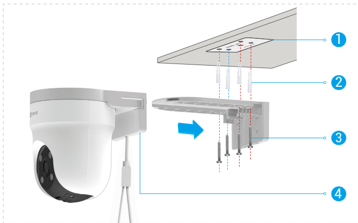
圖 1 天花板安裝
