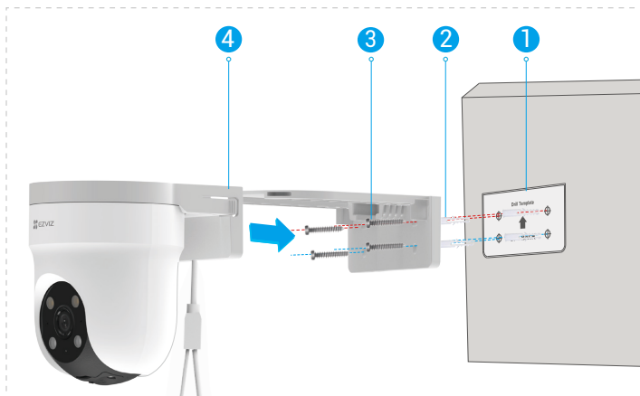
圖 2 壁掛式安裝
